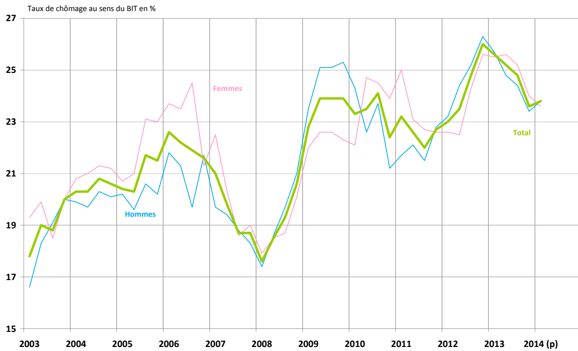
Graphique 13 : Taux de chômage des jeunes en France
